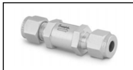
Rückschlagventil für Rohr OD 1/4", Öffnungsdruck 0,69 bar, Edelstahl 316
